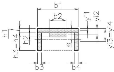
断面特性算出表
